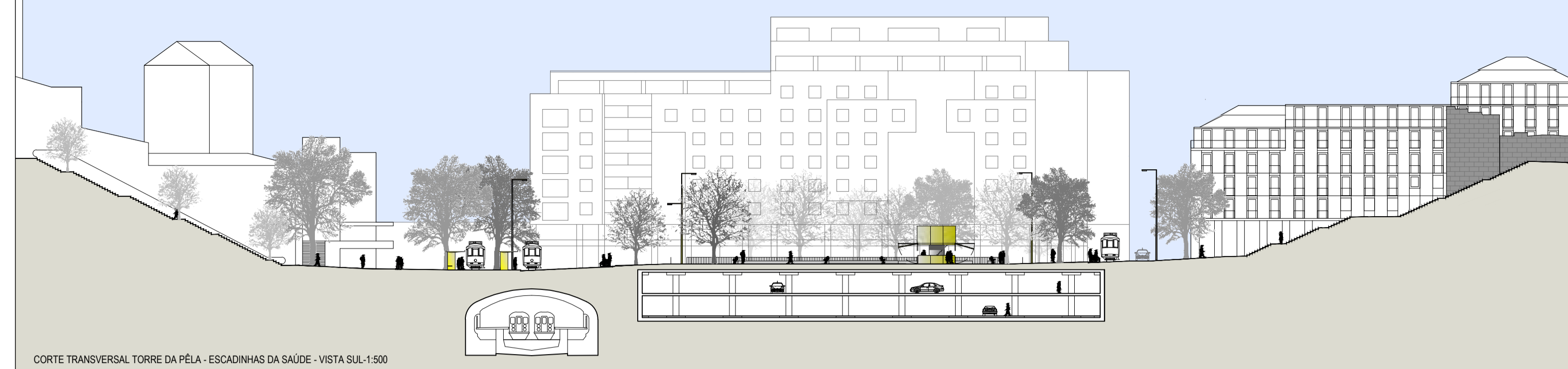
CORTE TRANSVERSAL TORRE DA PÉLA - ESCADINHAS DA SAÚDE - VISTA SUL-1:500
