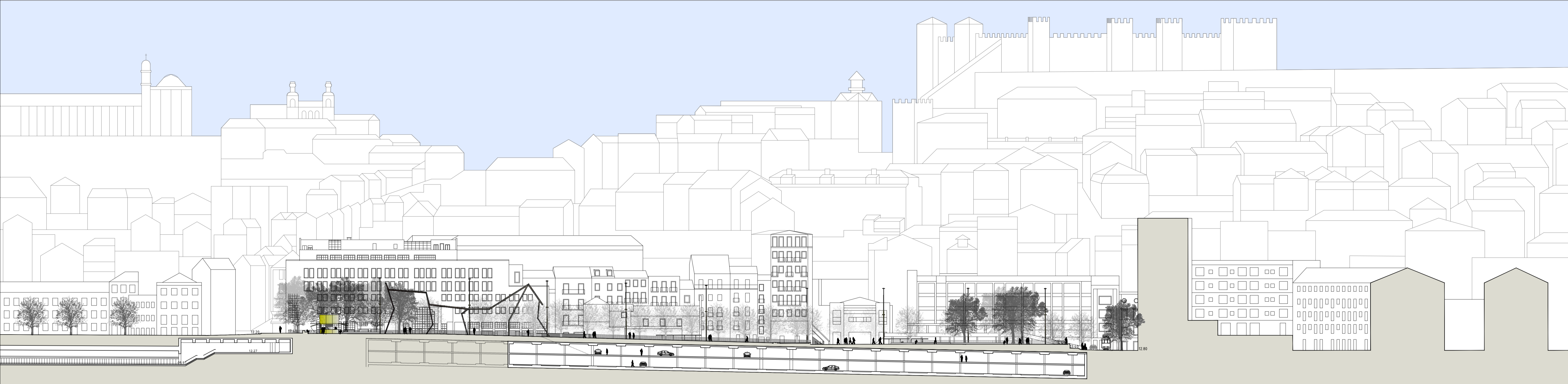
CORTE LONGITUDINAL NORTE-SUL ESCALA 1:500
