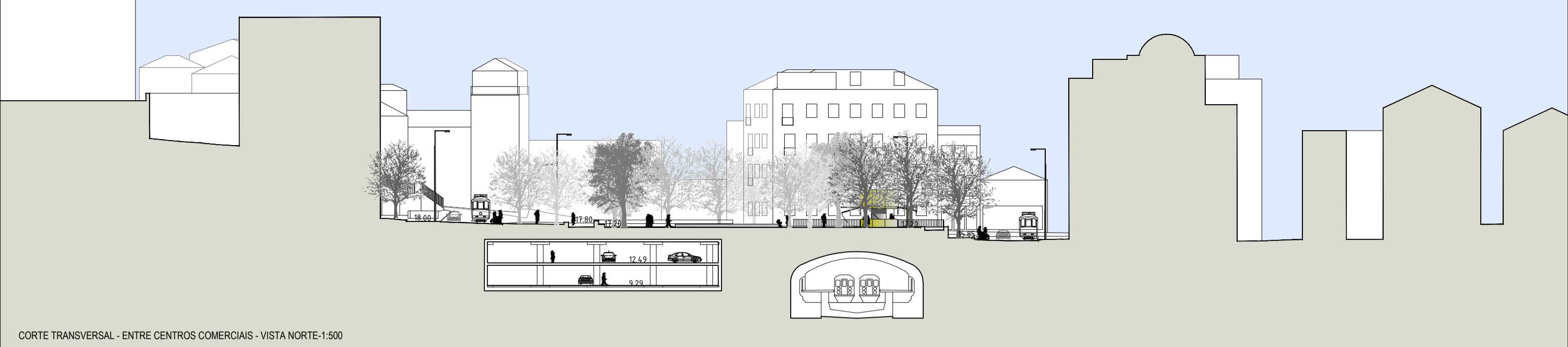
CORTE TRANSVERSAL - ENTRE CENTROS COMERCIAIS - VISTA NORTE-1:500
